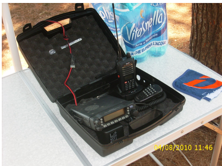
Radio da campo alimentata dalla batteria 12V dell'auto
